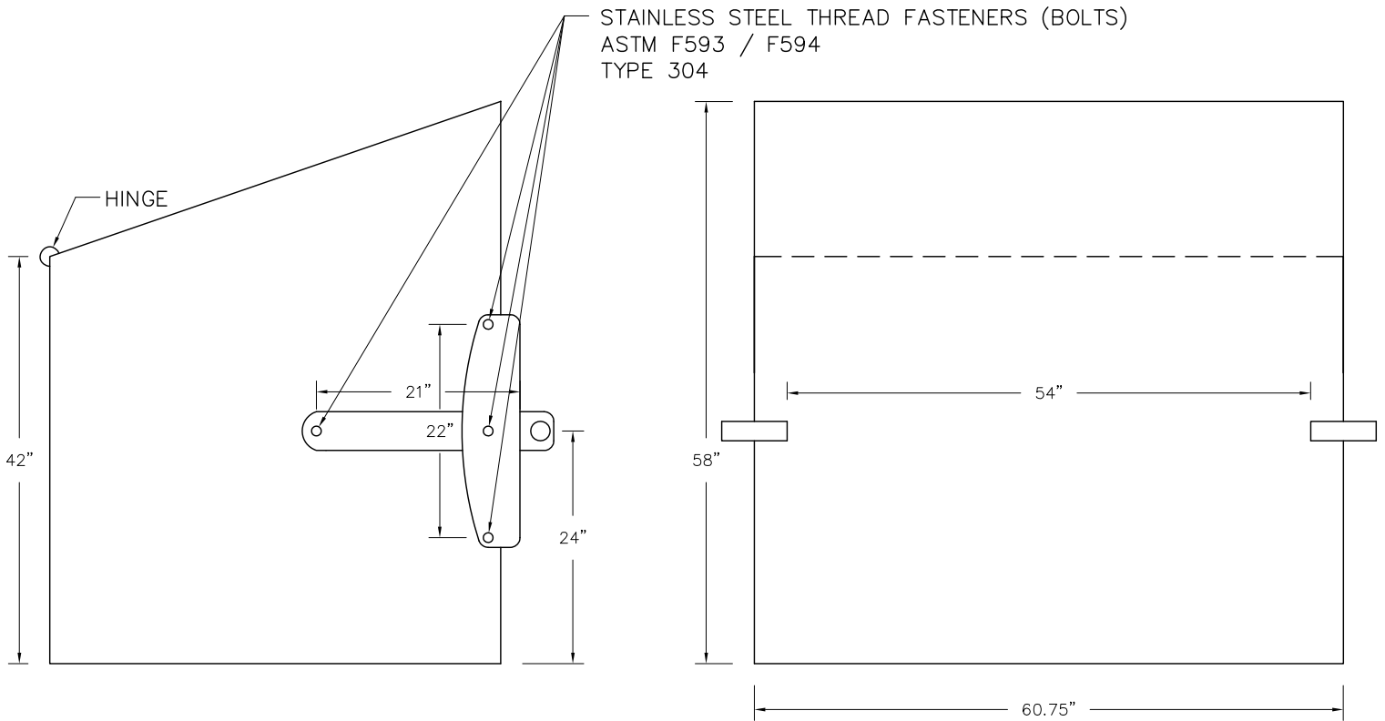
SIDE-LOAD CONTAINER SIDE N.T.S
